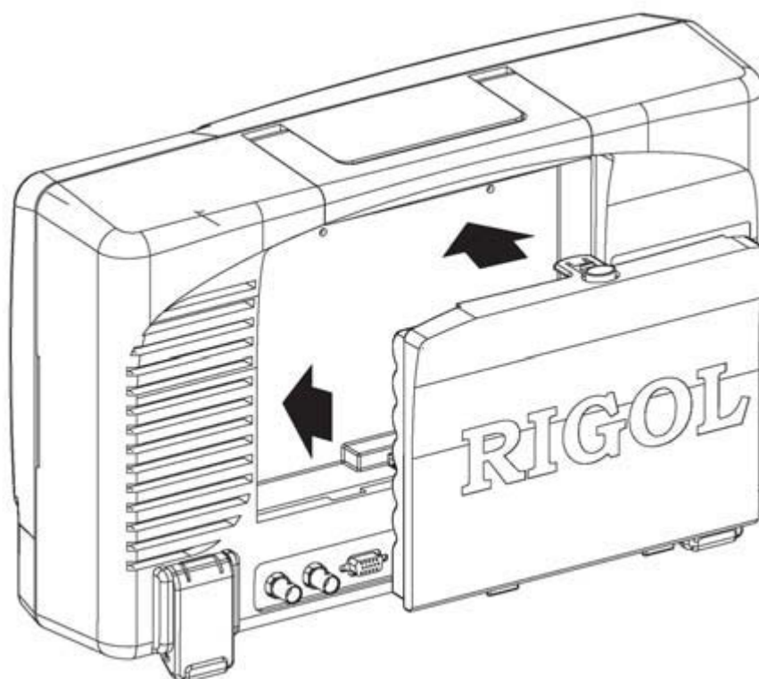
Рис. 1-6 Установка аккумулятора
